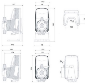
Dimensions Pompe Doseuse
